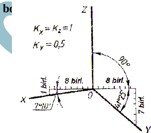
10-shakl. To'g'ri burchakli dimetrik
