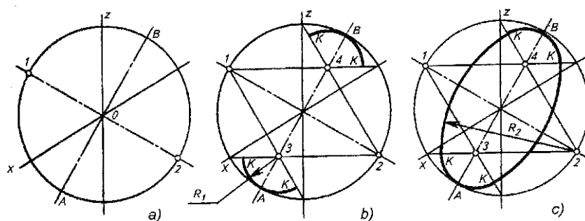
7-shakl. To'g'ri burchakli izometriyada ellips o'rniga oval yasash (1-usul)
