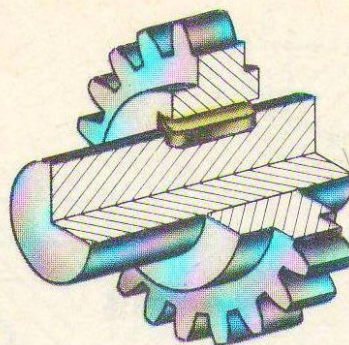
Шпонка призматическая обыкновенная ГОСТ 23360-78 (СТ СЭВ 189-75)
