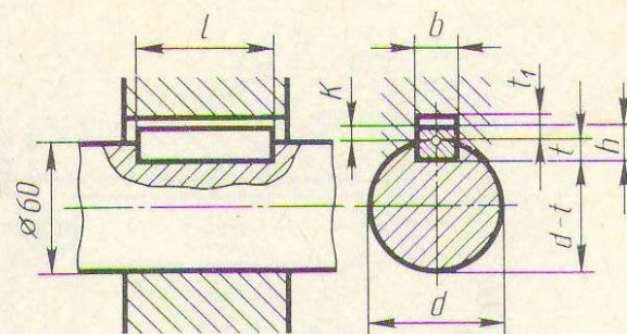
Шпонка призматическая обыкновенная ГОСТ 23360-78 (СТ СЭВ 189-75)
