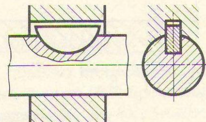
Шпонка сегментная ГОСТ 24071-80 (СТ СЭВ 647-77)
