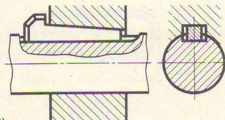
Шпонка клиновья ГОСТ 24063-80 (СТ СЭВ 645-77)
