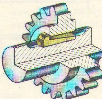
Шпонка клиновья ГОСТ 24063-80 (СТ СЭВ 645-77)
