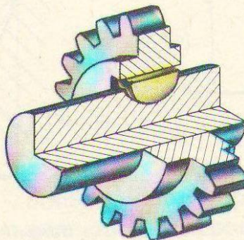
Шпонка сегментная ГОСТ 24071-80 (СТ СЭВ 647-77)
